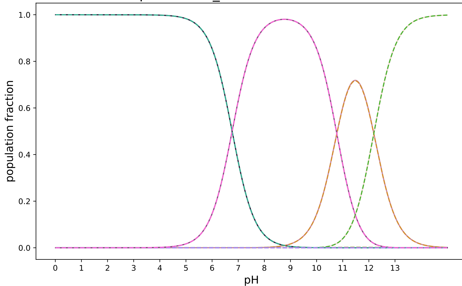
pKa-3DS-1_modified:SAMPL8-16
