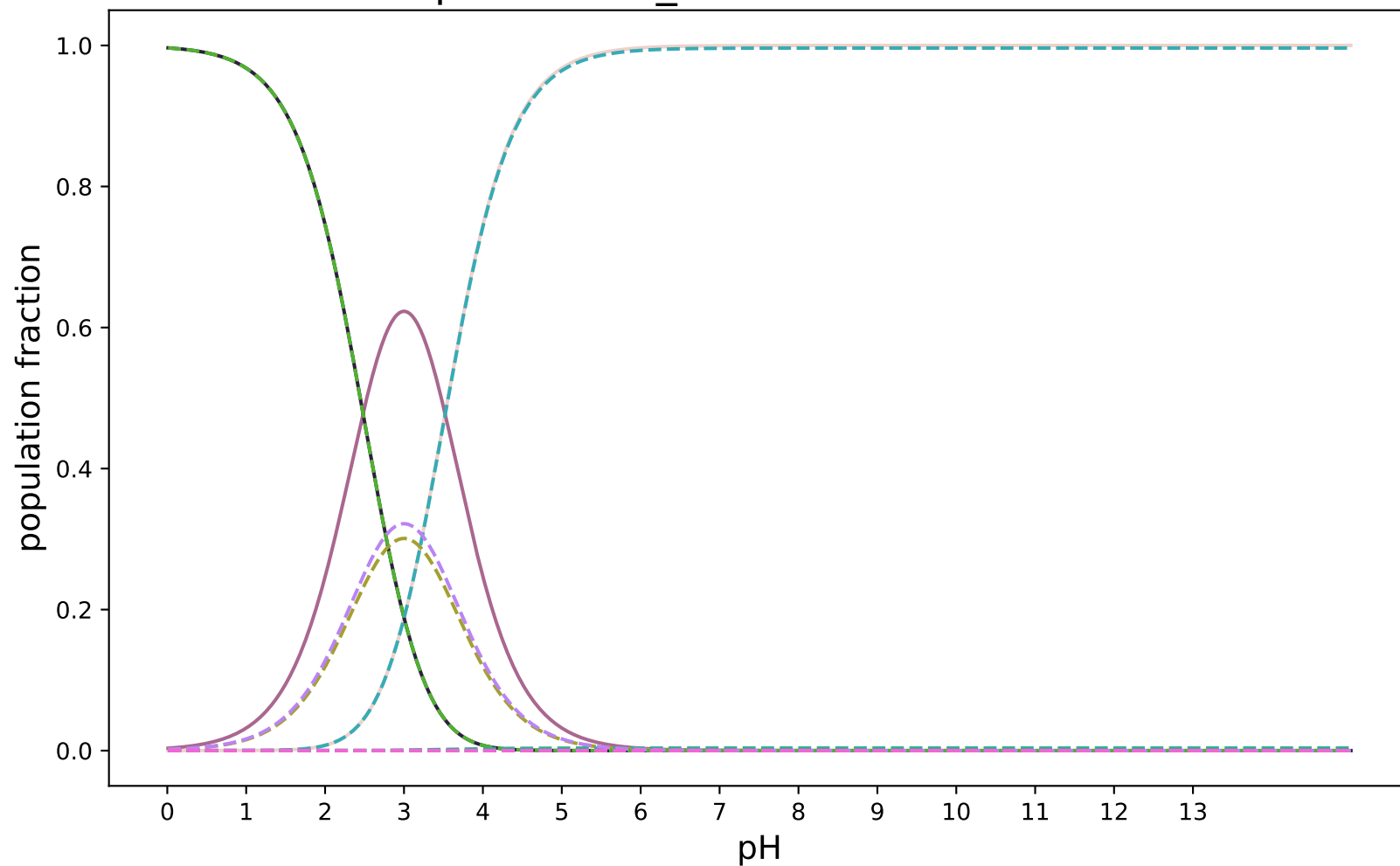
pKa-3DS-1 modified:SAMPL8-4
