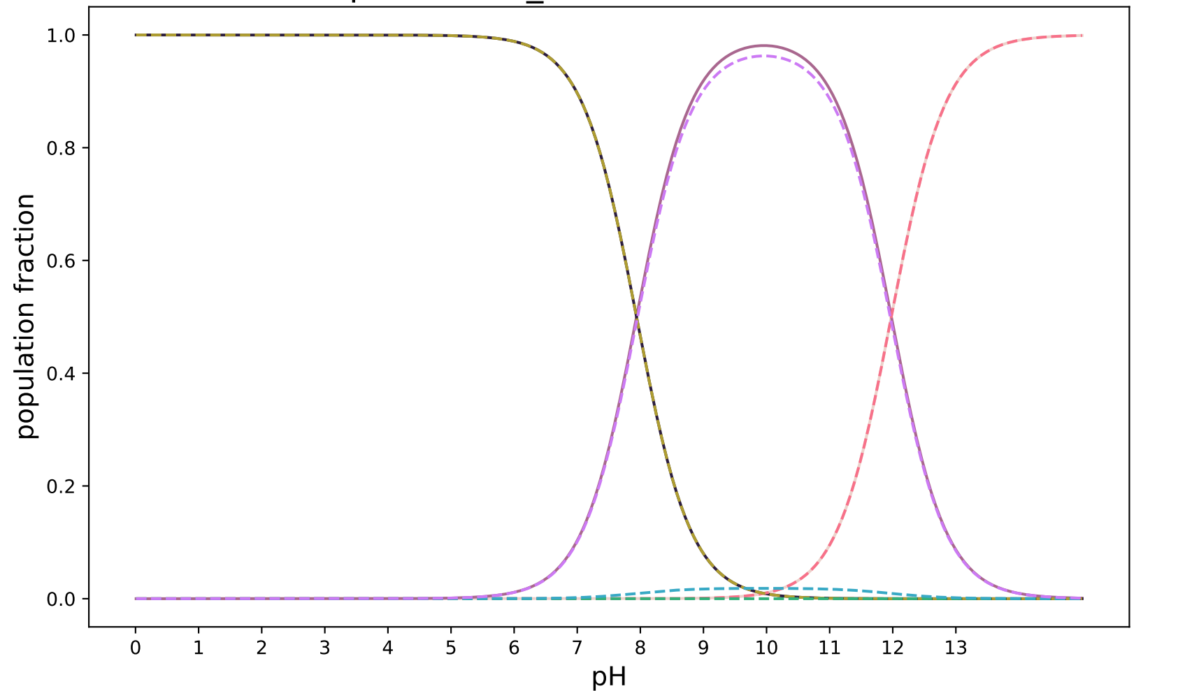
pKa-3DS-1_modified:SAMPL8-7
