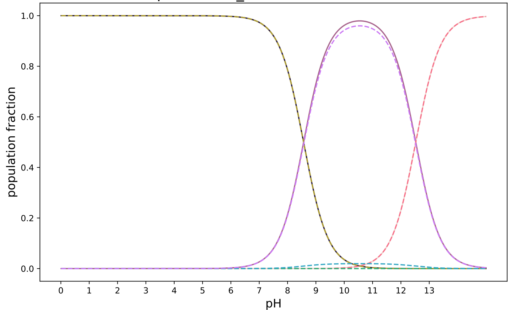
pKa-3DS-3_modified:SAMPL8-7
