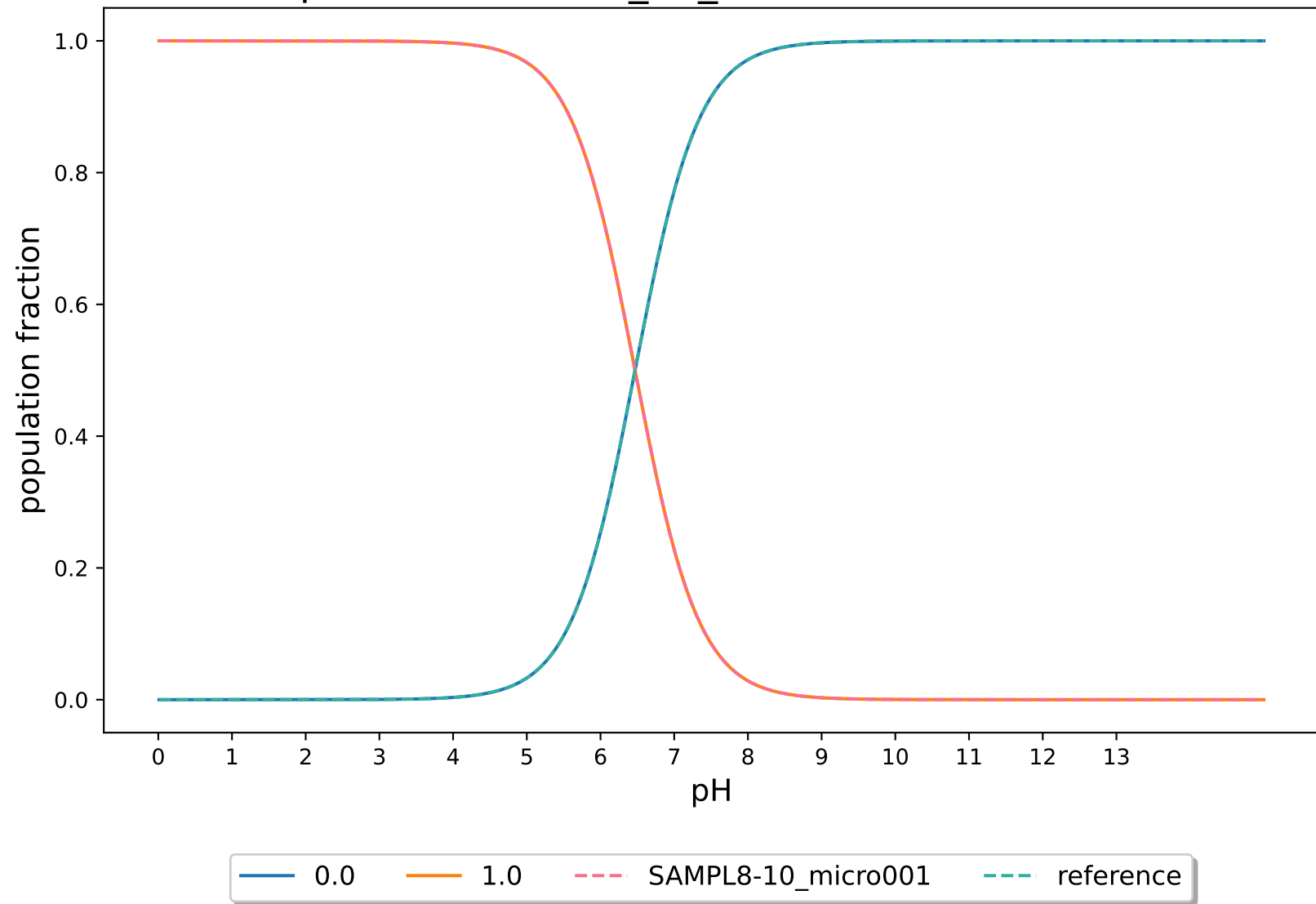
pKa-RobertRaddi_RF_modified:SAMPL8-10
