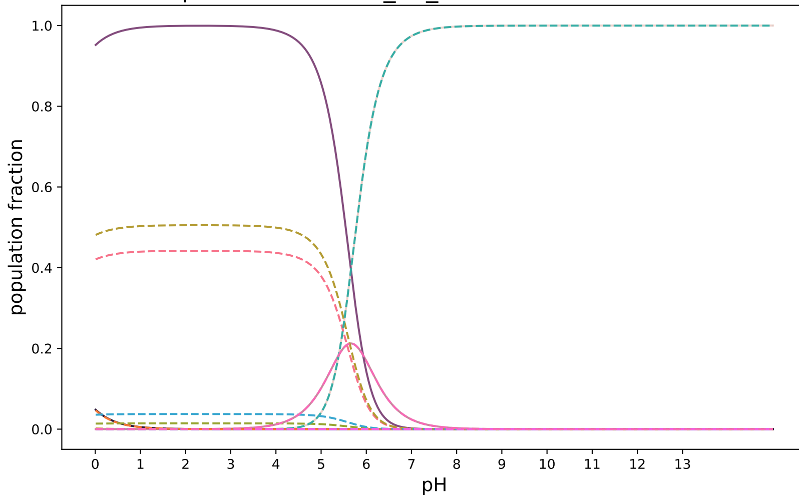
pKa-RobertRaddi_RF_modified:SAMPL8-19
