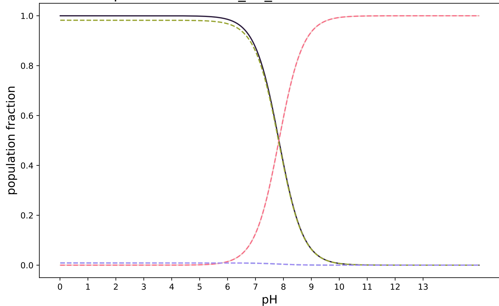
pKa-RobertRaddi_RF_modified:SAMPL8-22
