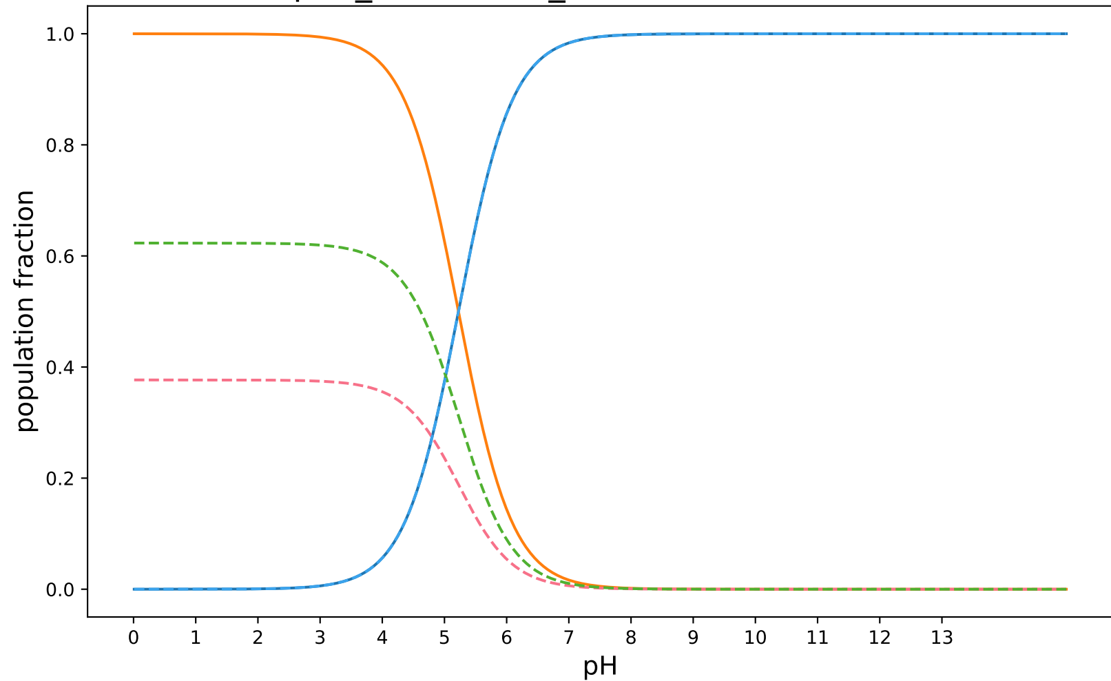
pKa_Chemaxon_modified:SAMPL8-12
