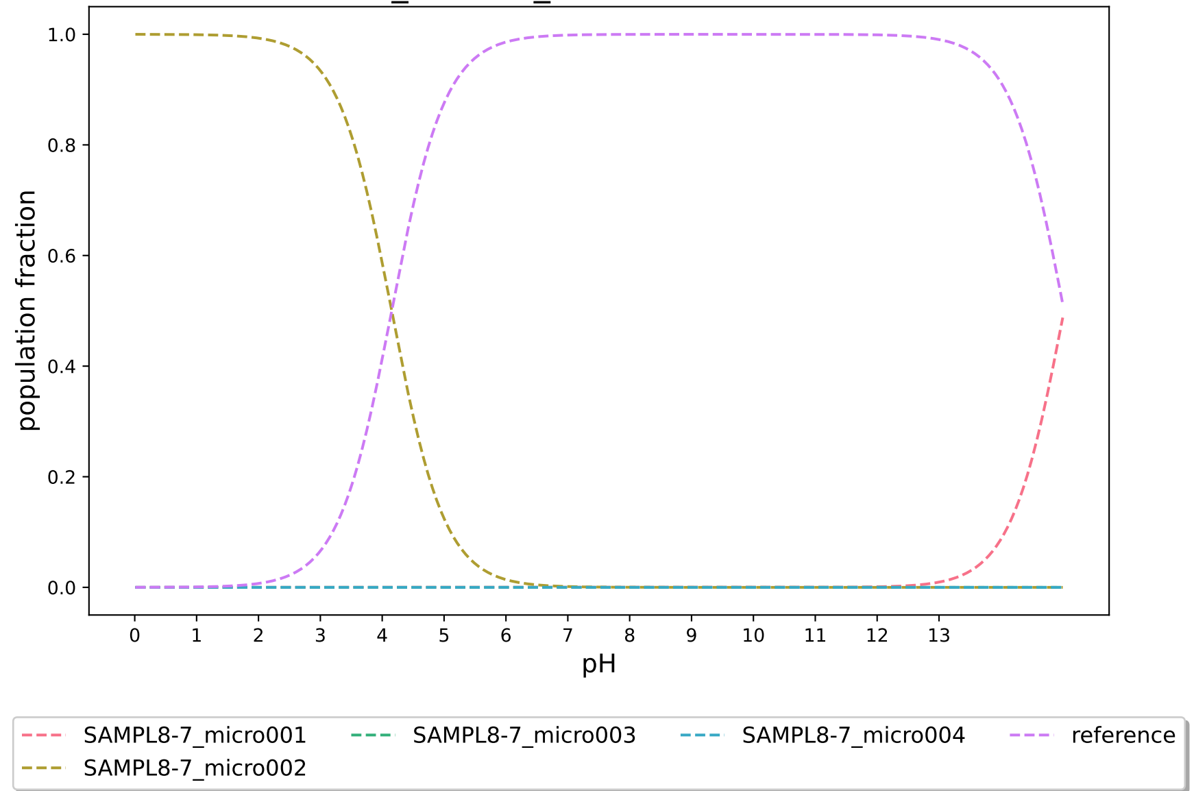
PKA_ECRISM_modified:SAMPL8-7
