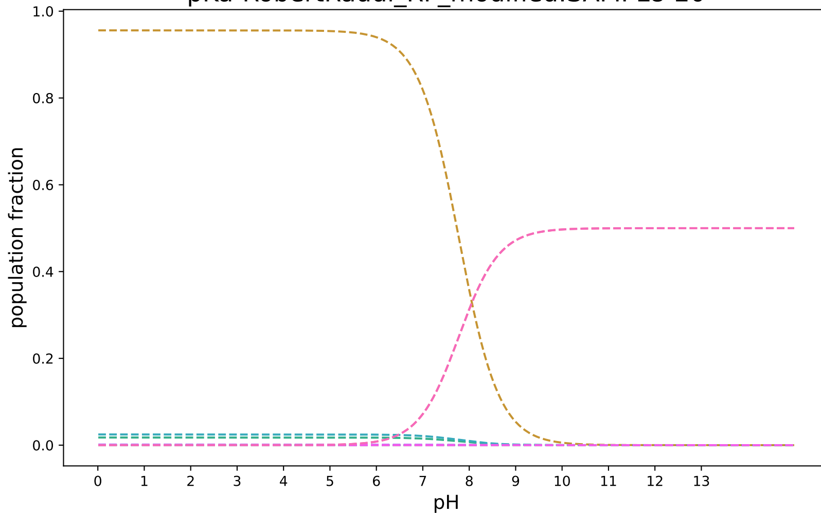
pKa-RobertRaddi_RF_modified:SAMPL8-20
