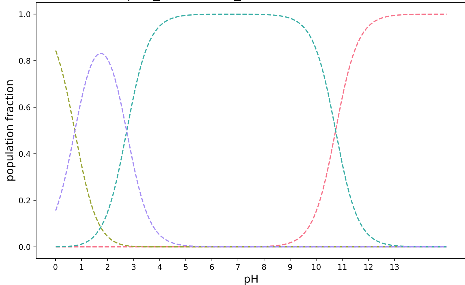
pKa_Chemaxon_modified:SAMPL8-4
