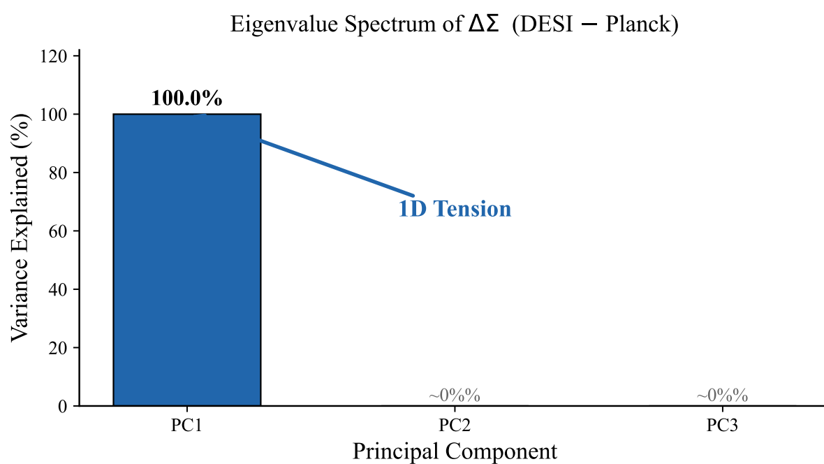
图 2: B-算子 \mathcal{B} = \Sigma_P^{-1/2}(\Sigma_P - \Sigma_{PD})\Sigma_P^{-1/2} 的特征值谱。PC1 捕获了总协方差收缩的 > 99.99\% 。所有更高阶 PCs 的特征值均与零无法区分。张力是严格一维的。
