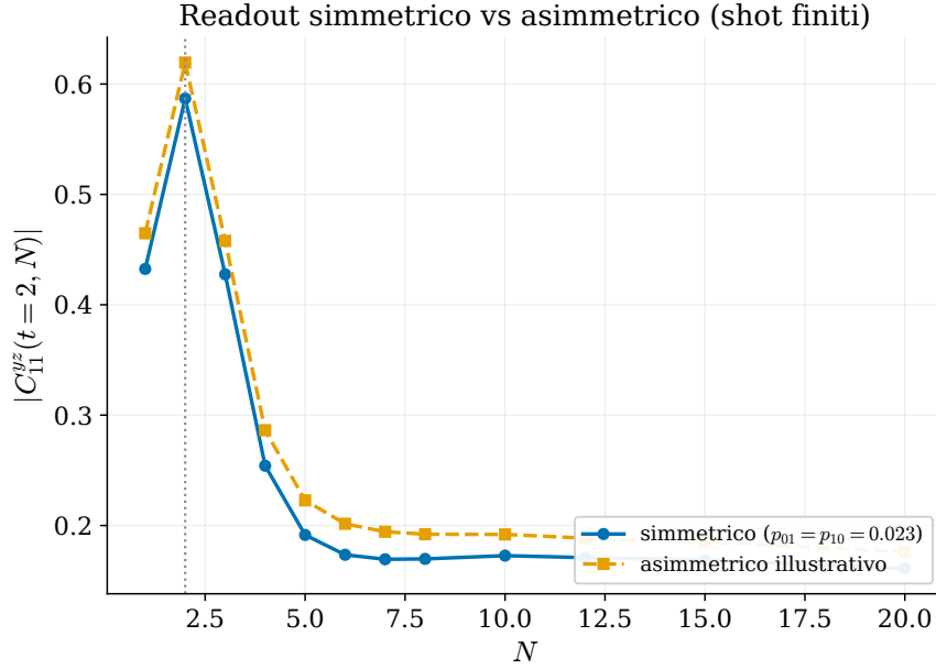
Figura 1: Modulo del correlatore rumoroso |C_{11}^{yz}(t=2, N)| in funzione di N , readout genuinamente campionato: simmetrico ( p_{01} = p_{10} = 0.023 ) contro asimmetrico ( p_{01} = 0.0115 , p_{10} = 0.0345 , stessa media). Il massimo resta a N^* = 2 in entrambi i casi. Lo split asimmetrico alza |C(N)| su tutti gli N testati, non solo a N grande: l’offset \beta(1+i) si somma qui in modo costruttivo con C_{ideale}(N) su tutto l’intervallo — non un effetto casuale, ma dipendente dalla fase specifica di C_{ideale}(N) per questo problema.
