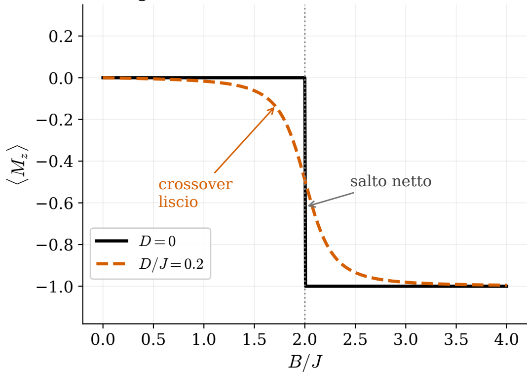
Magnetizzazione dello stato fondamentale
