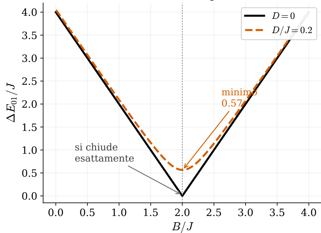
Distanza fondamentale-primo eccitato
