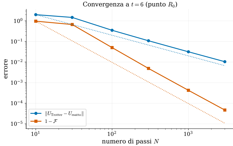
Figura 6: Errore a t = 6 (punto R_0 ), scala doppio-logaritmica. Le rette punteggiate sono le pendenze asymptotiche attese ( -1 per la norma dell'operatore, -2 per 1 - \mathcal{F} ).
