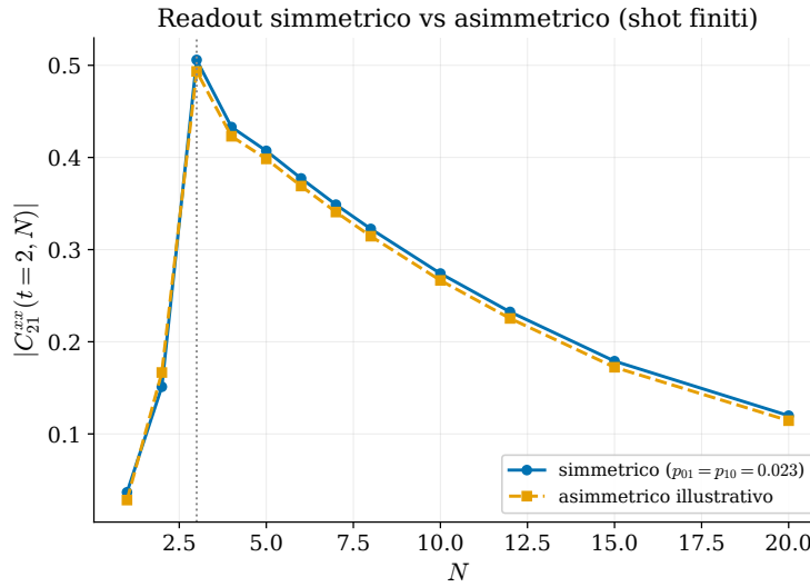
Figura 17: |C_{21}^{xx}(t=2, N)| , readout simmetrico contro asimmetrico ( 8 \times 10^4 shot per punto). N^* = 3 in entrambi i casi.
