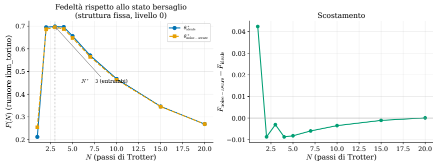
Figura 16: Fedeltà di Trotter, struttura fissa. N^* = 3 in entrambi i casi; scostamento piccolo, su scala \sim 10^{-2} .
