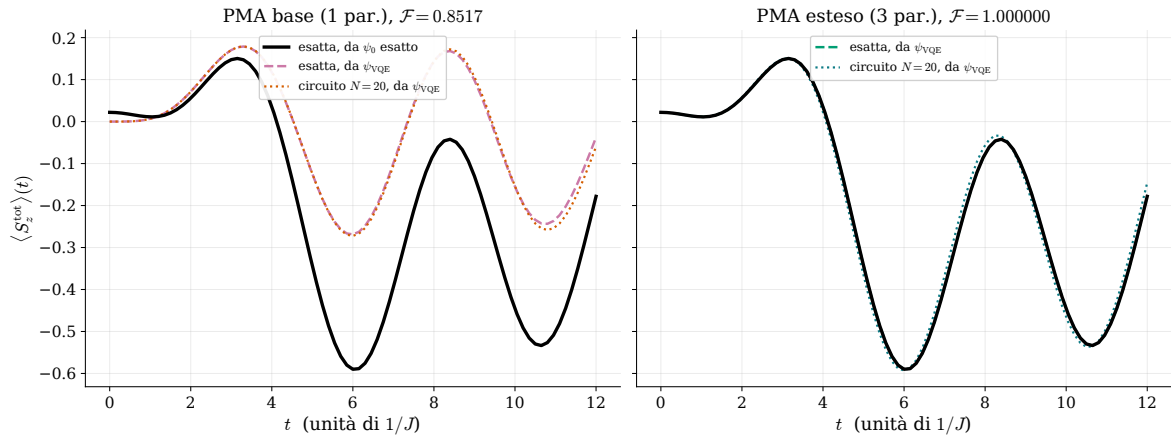
Figura 13: Evoluzione di \langle S_z^{\text{tot}} \rangle(t) al punto P2, con N = 20 passi di Trotter, a partire dai due ansatz del VQE. Nera: evoluzione esatta dal fondamentale esatto. Tratteggiata: evoluzione esatta a partire dallo stato del VQE (isola l'errore di preparazione). Punteggiata: evoluzione con il circuito di Trotter a partire dallo stesso stato (entrambi gli errori). Sinistra , PMA base: le curve del VQE si staccano nettamente dall'esatta. Destra , PMA esteso: le tre curve sono indistinguibili.
