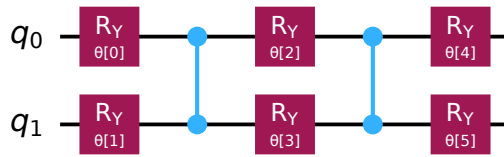
Figura 3: Ansatz generico hardware-efficient: rotazioni R_y alternate a porte CZ , 6 parametri.
