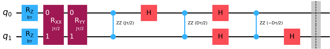
Figura 10: Struttura simbolica di un passo di Trotter: stessa sequenza di porte della Fig. 11, con gli angoli espressi in funzione di J, b, D, \tau anziché nei valori numerici di un punto di lavoro specifico.
