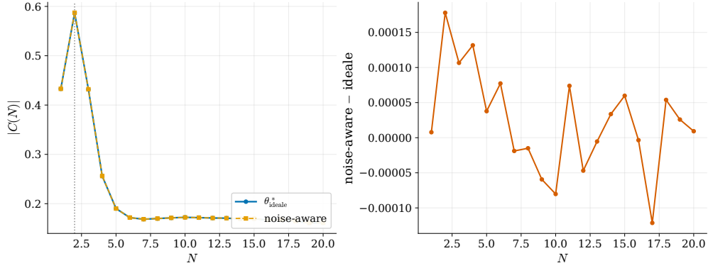
Figura 26: Modulo del correlatore rumoroso, riuso ideale contro noise-aware: massimo a N^* = 2 in entrambi i casi.
