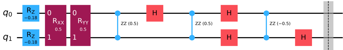
Figura 11: Un singolo passo di Trotter: e^{-iH_1\tau} (rotazioni R_z del campo, poi R_{xx}, R_{yy}, R_{zz} dello scambio) seguito da e^{-iH_2\tau} (termine DM, due R_{zz} coniugate da Hadamard). Il circuito completo è questo blocco ripetuto N volte.
