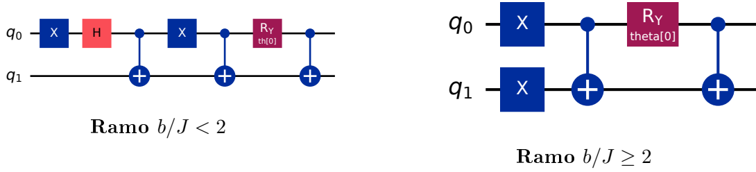
Figura 5: Ansatz PMA base nei suoi due rami: preparazione del singoletto (sinistra) o di |11\rangle (destra), seguita dallo stesso blocco parametrico di Fig. 4.
