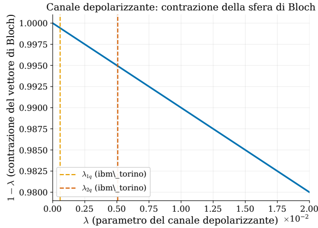
Figura 18: Contrazione del vettore di Bloch, 1 - \lambda , in funzione di \lambda . Ai valori di calibrazione di riferimento la contrazione è piccola (sotto l'1%) ma non nulla.
