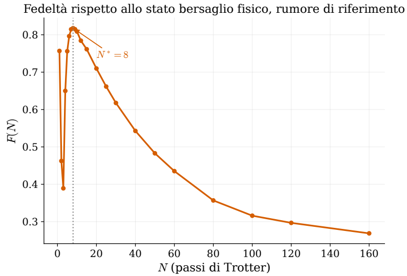
Figura 20: Fedeltà F(N) rispetto allo stato bersaglio fisico, a rumore di riferimento. Crescita rapida per N piccolo (l'errore di Trotter domina), massimo a N^* = 8 , decrescita lenta per N grande (il rumore di gate accumulato domina).
