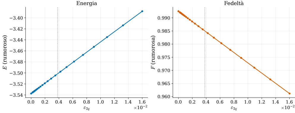
Figura 19: Energia e fedeltà rumorose in funzione di \varepsilon_{2q} , a \varepsilon_{1q} e p_{\text{readout}} fissati al valore di riferimento (linea tratteggiata). Degradazione monotona, nessuna soglia.
