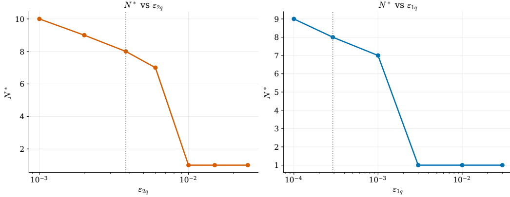
Figura 24: N^* (fedeltà di Trotter) in funzione di \varepsilon_{2q} (sinistra) e \varepsilon_{1q} (destra), scala log. Monotonia non-crescente, con transizione a N^* = 1 per rumore sufficientemente forte.
