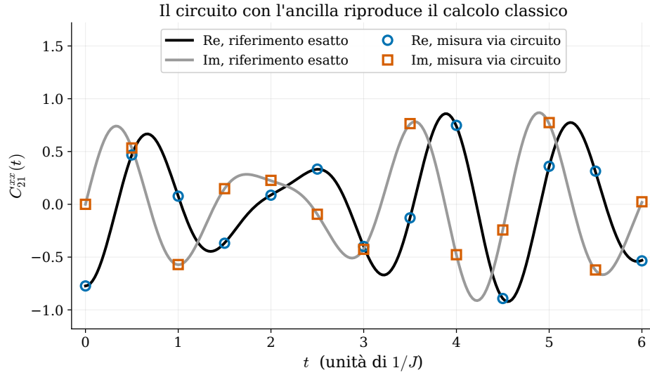
Figura 15: Correlatore rappresentativo su t \in [0, 6] : curve continue (riferimento numerico esatto, esponenziale di matrice diretto a precisione di macchina) contro il circuito quantistico, parte reale e immaginaria.
