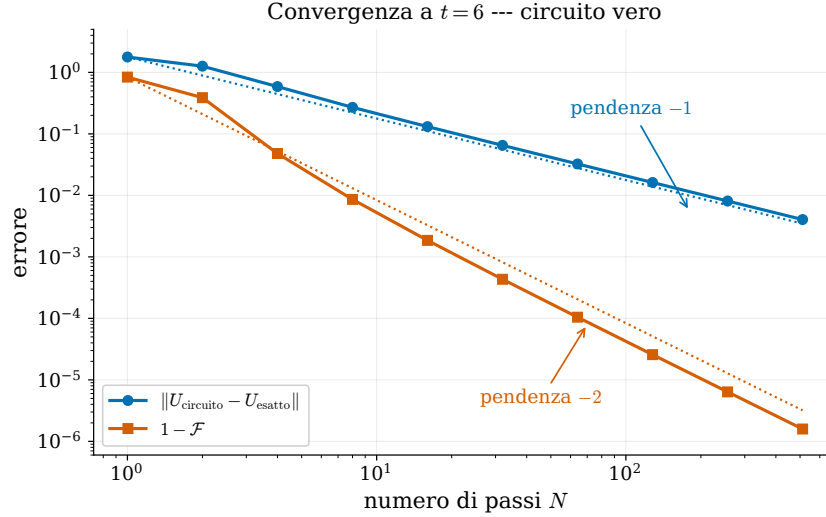
Figura 12: Errore a tempo fissato ( t = 6 ) al crescere di N , scala doppio-logaritmica: distanza fra operatori di evoluzione (blu, scaling 1/N ) e perdita di fidelity sullo stato (rosso, scaling 1/N^2 ). Le rette tratteggiate sono le pendenze teoriche attese.
