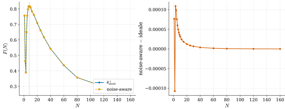
Figura 25: Fedeltà di Trotter F(N) , riuso ideale contro noise-aware: massimo a N^* = 8 in entrambi i casi; lo scostamento (pannello destro, scala ingrandita) resta \sim 10^{-4} .
