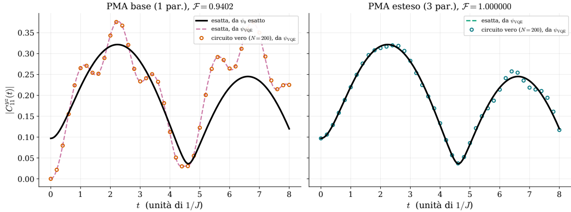
Figura 17: |C_{11}^{yz}(t)| su t \in [0, 8] , preparato con i due ansatz e fatto evolvere con il circuito completo. Sinistra , PMA base: scarto visibile dal riferimento esatto. Destra , PMA esteso: curve pressoché indistinguibili.
