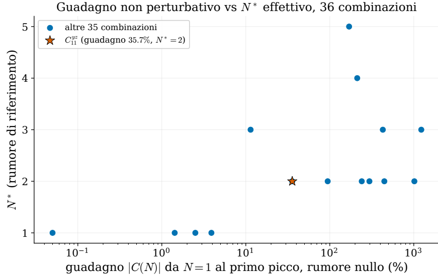
Figura 23: Relazione fra il guadagno di |C(N)| da N = 1 al primo picco (rumore nullo) e il valore di N^* effettivo sotto rumore di riferimento, sulle 36 combinazioni. Le combinazioni con guadagno trascurabile ( \lesssim 10\% ) collassano quasi tutte a N^* = 1 — nessun compromesso da negoziare. Al crescere del guadagno, N^* tende a salire. C_{11}^{yz} (guadagno 35.7%, N^* = 2 ) cade a metà della distribuzione, non in un estremo — coerente con la sua scelta come caso rappresentativo. La relazione non è perfettamente monotona punto per punto, ma la tendenza di fondo è chiara.
