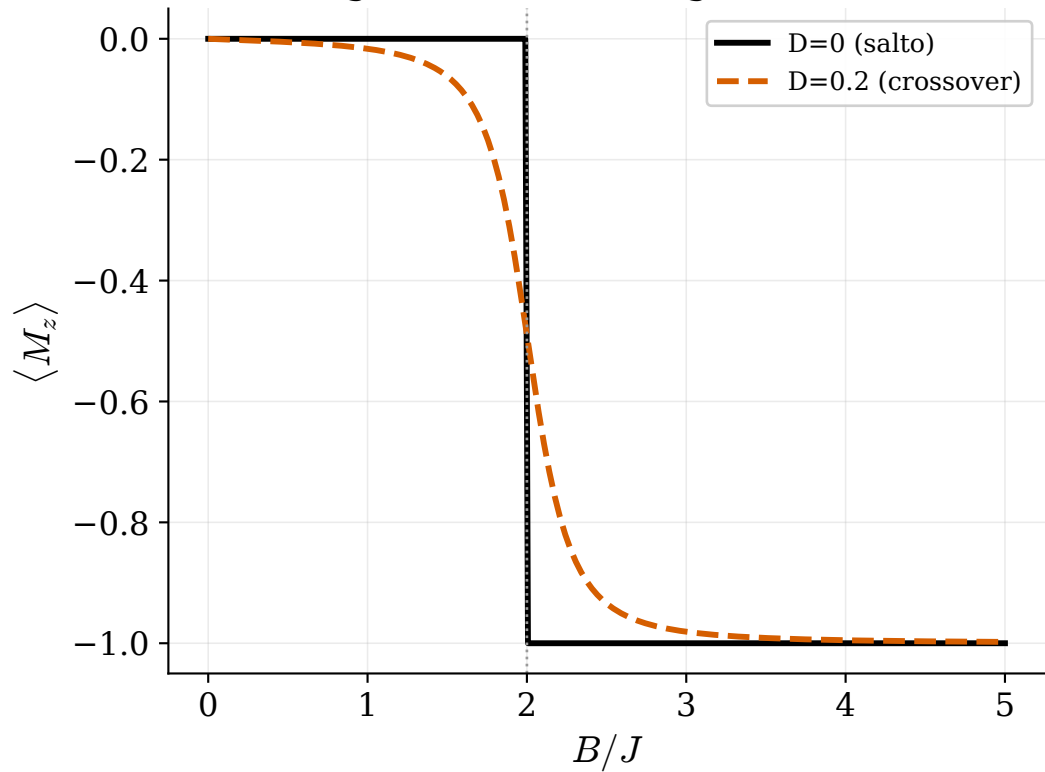
Magnetizzazione del ground state
