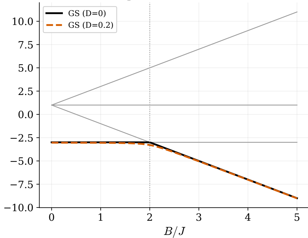
Spettro del dimero
