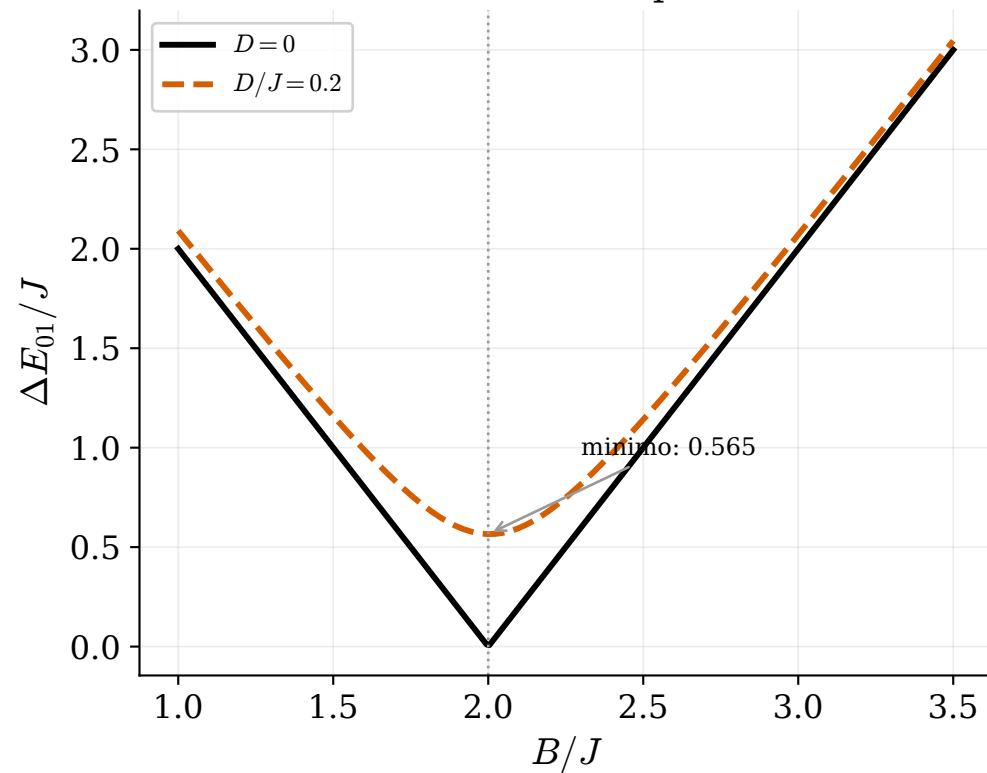
Distanza fondamentale-primo eccitato
