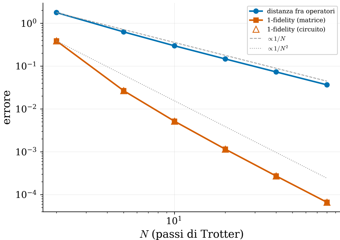
Error e a t = 6 , matrice e circuito
