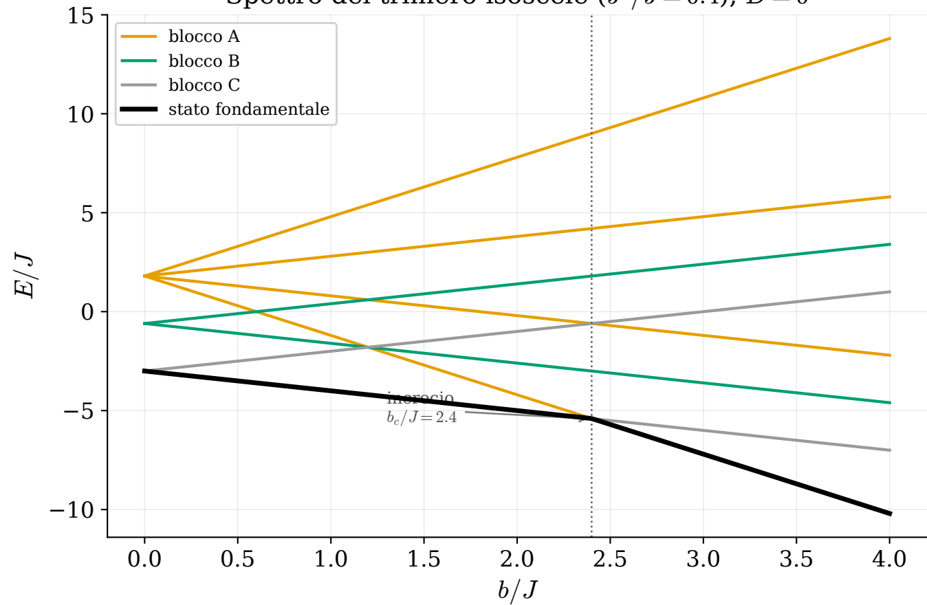
Spettro del trimero isoscele ( J'/J=0.4 ), D=0
