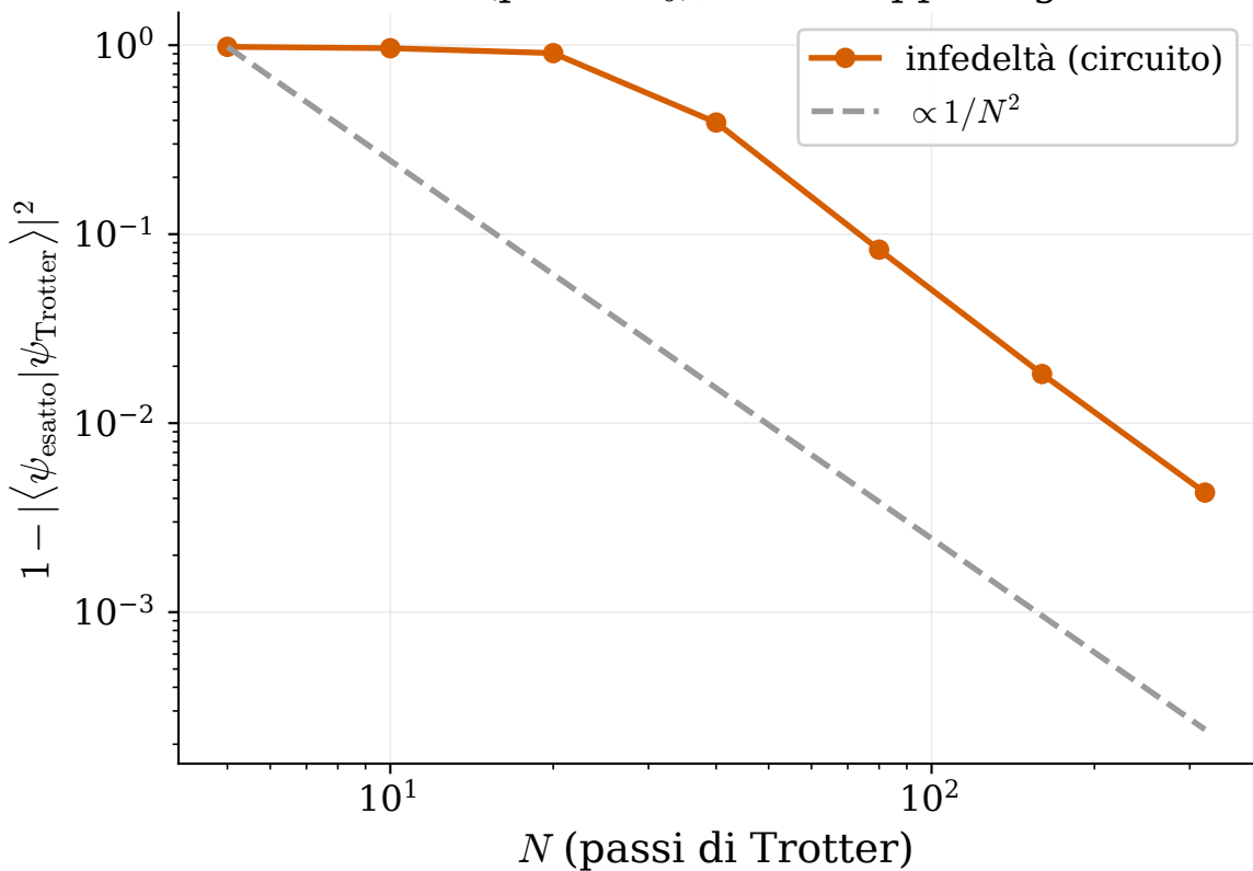
Errore a t = 6 (punto R_0 ), scala doppio-logaritmica
