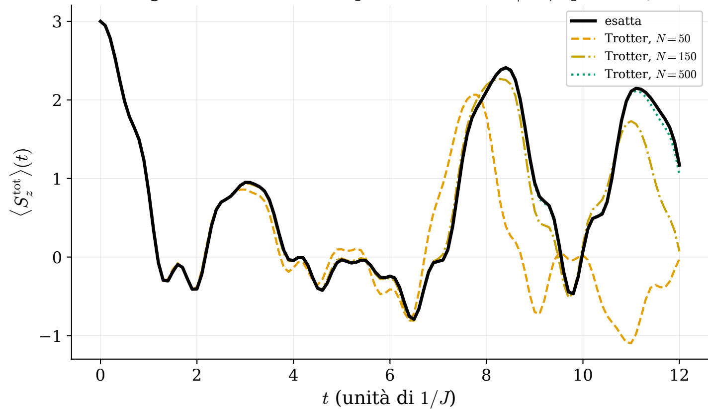
Magnetizzazione nel tempo, stato iniziale |000\rangle (punto R_0 )
