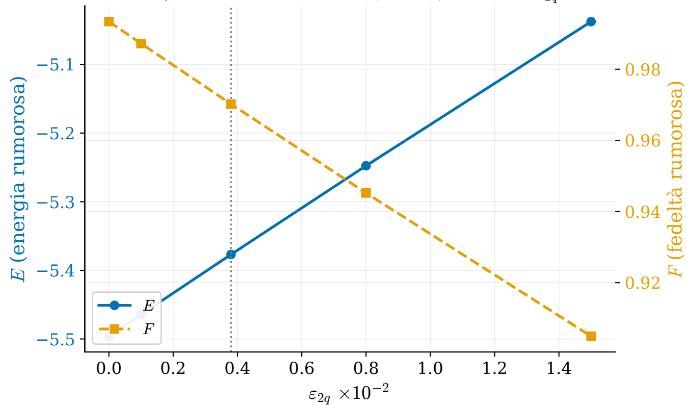
VQE+DM sotto rumore (anello): scan su \varepsilon_{2q}
