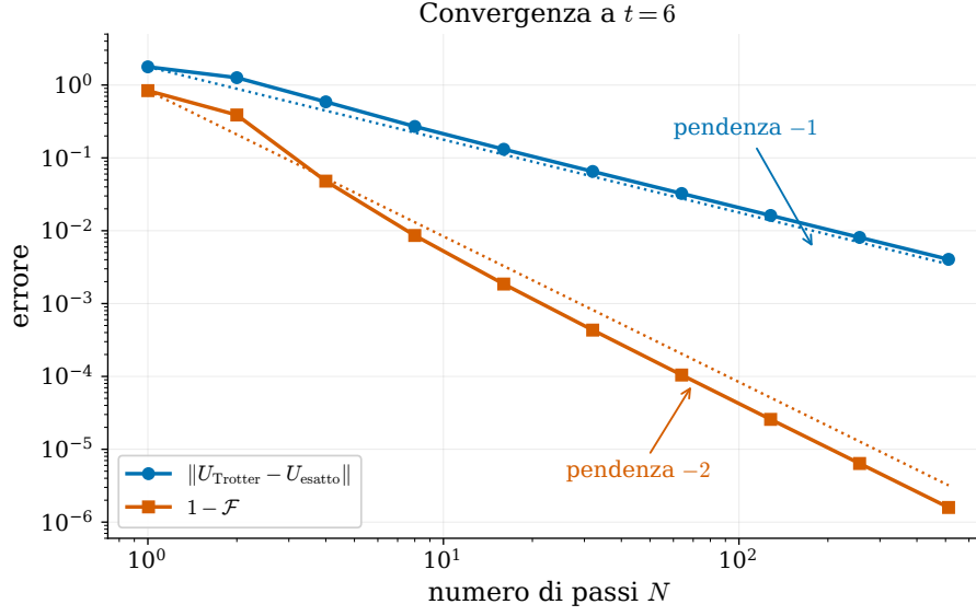
Figura 4: Errore a tempo fissato ( t = 6 ) al crescere del numero di passi, in scala doppio-logaritmica. Le due grandezze misurano cose diverse: la distanza fra gli operatori di evoluzione (blu) scala come 1/N , la perdita di fidelity sullo stato (rosso) come 1/N^2 . Le rette punteggiate sono le pendenze attese, ancorate al primo punto. Gli scostamenti a N piccolo sono i termini di ordine superiore, che a pochi passi non sono trascurabili.
