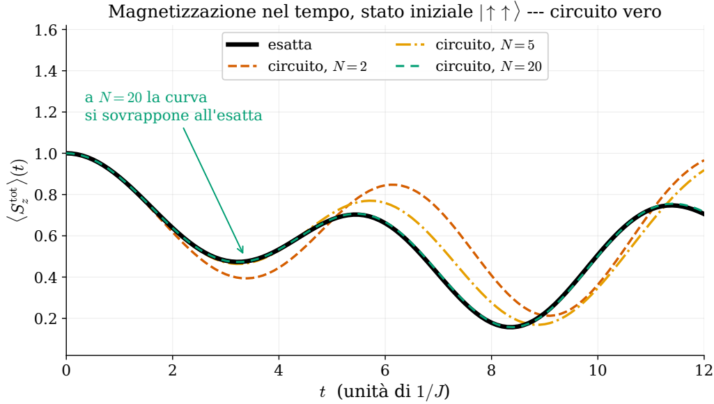
Figura 3: Circuito vero: stesso passo di Fig. 1, transpilato in porte native, composto N volte. Stesso punto di lavoro, stesso stato iniziale, stessi valori di N della Fig. 2. Il punto di lavoro è scelto perché la dinamica non sia monocromatica: un'unica frequenza renderebbe l'errore molto più difficile da vedere.
