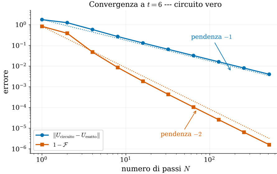
Figura 5: Stesso identico calcolo di Fig. 4, ma con il circuito vero (transpilato, eseguito porta per porta) per ciascuno dei 10 valori di N , al posto della matrice compatta.
