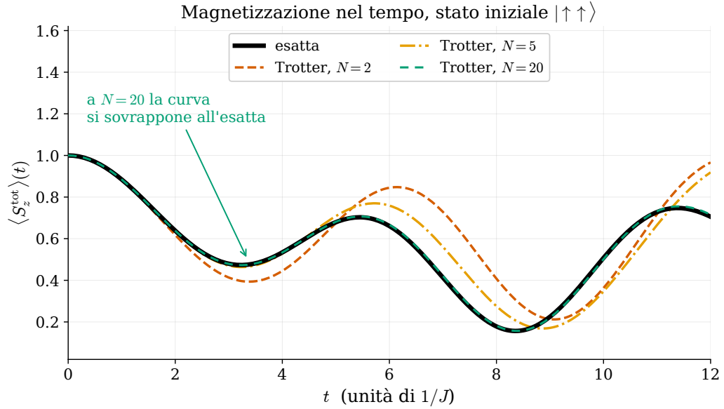
Figura 2: Matrice compatta (e^{-iH_2\tau}e^{-iH_1\tau})^N , algebra lineare diretta, nessuna porta applicata. La curva nera è l'evoluzione esatta. Con soli 2 passi (rosso) l'approssimazione sbaglia visibilmente ampiezza e fase; con 5 passi (arancio) l'errore si riduce ma resta; con 20 passi (verde) la curva si sovrappone all'esatta.
