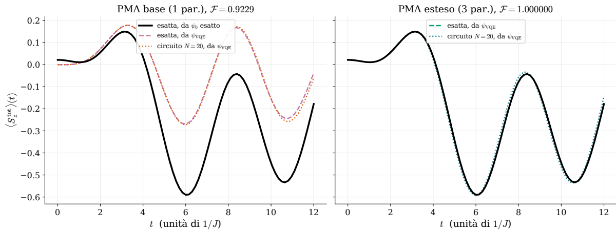
Figura 6: Stesso punto di lavoro, stesso trattamento, due ansatz diversi dal Documento 2. In entrambi i pannelli: nera, l'evoluzione esatta dal fondamentale esatto (il riferimento); tratteggiata, evoluzione esatta ma a partire dallo stato del VQE (isola l'errore di preparazione); punteggiata, evoluzione con il circuito ( N = 20 passi di Trotter) dallo stesso stato del VQE (entrambi gli errori insieme). A sinistra , PMA base: le due curve del VQE si staccano nettamente da quella esatta. A destra , PMA esteso: tutte e tre le curve sono indistinguibili a occhio.
