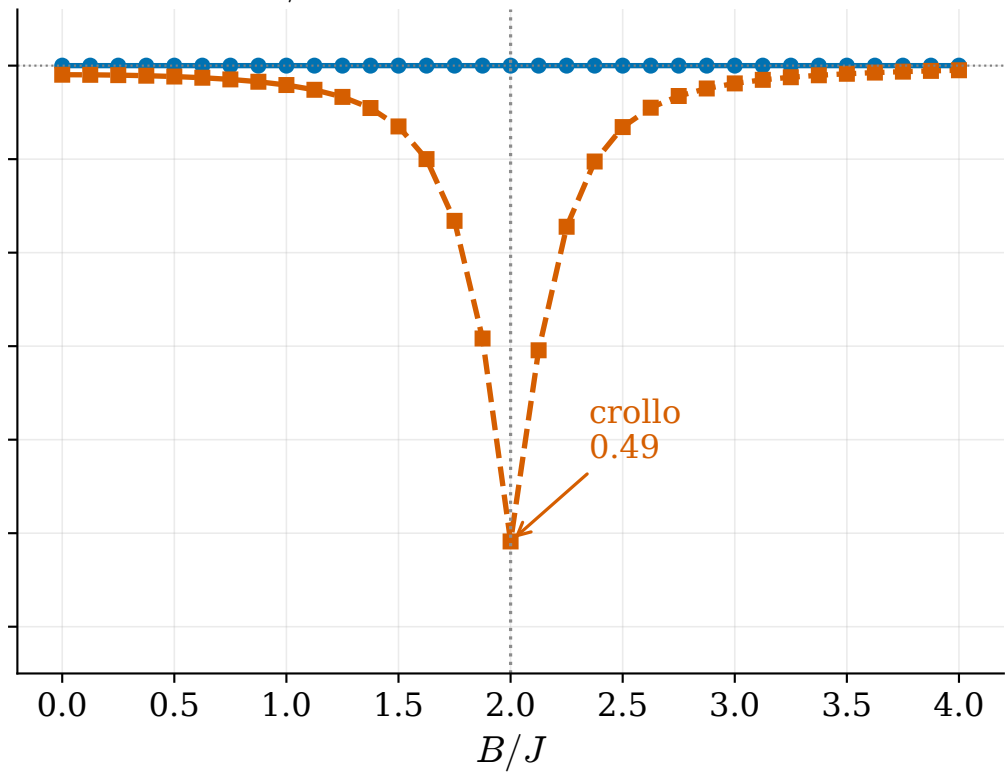
D/J=0.2 (simmetria rotta)
