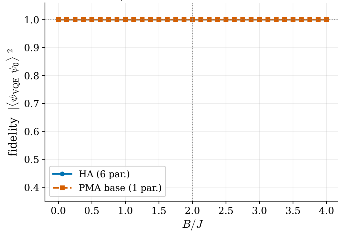
D/J=0.0 (simmetria intatta)
