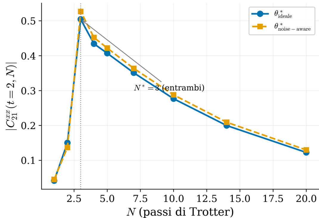
Correlatore rumoroso: ideale vs noise-aware (struttura fissa, livello 0)
