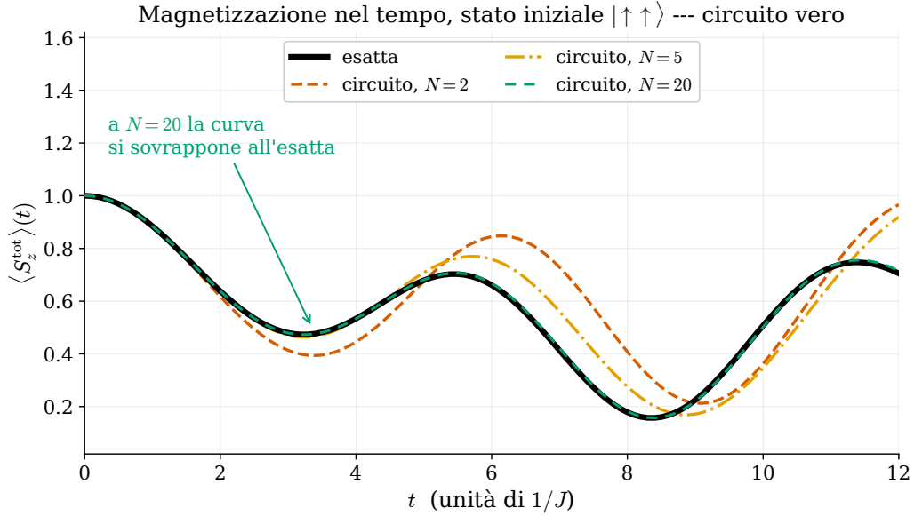
Figura 3: Circuito vero : stesso passo di Fig. 1, transpilato in porte native, composto N volte. Stesso punto di lavoro, stesso stato iniziale, stessi valori di N della Fig. 2. Il punto di lavoro è scelto perché la dinamica non sia monocromatica: un'unica frequenza renderebbe l'errore molto più difficile da vedere.
