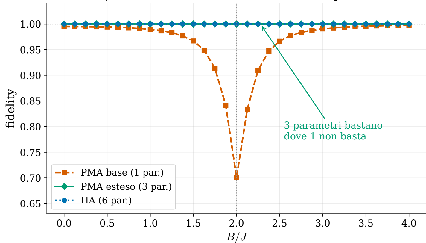
D/J=0.2 — effetto delle rotazioni che rompono M
