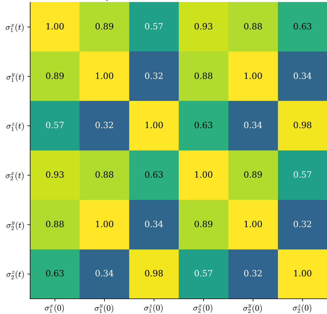
\max_t |C_{ij}^{\alpha\beta}(t)| (esatto, riferimento)
