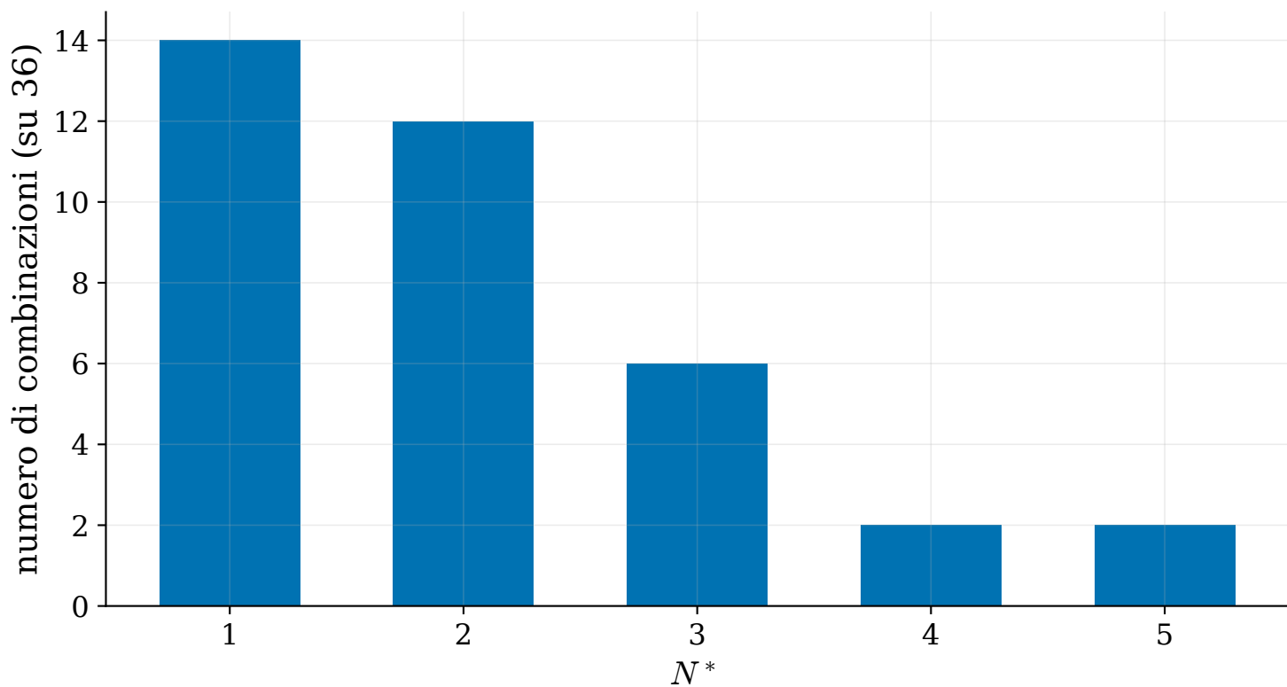
Tutte le 36 curve, readout a shot finiti
