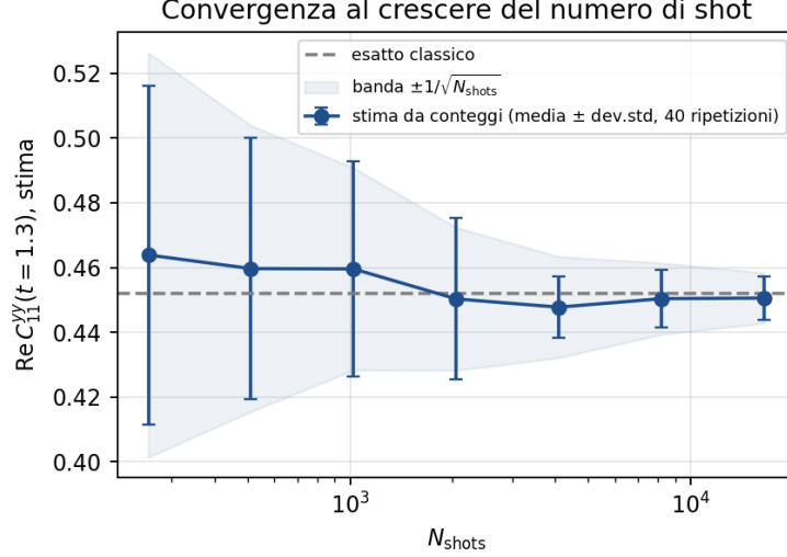
Figura 4: Stima di \text{Re } C_{11}^{yy}(t=1.3) al crescere del numero di shot (media e deviazione standard su 40 ripetizioni indipendenti del campionamento, N=200 passi di Trotter). La banda ombreggiata è \pm 1/\sqrt{N_{\text{shots}}} . La dispersione si restringe coerentemente con la soglia statistica attesa; la media converge al valore esatto classico (linea tratteggiata).
