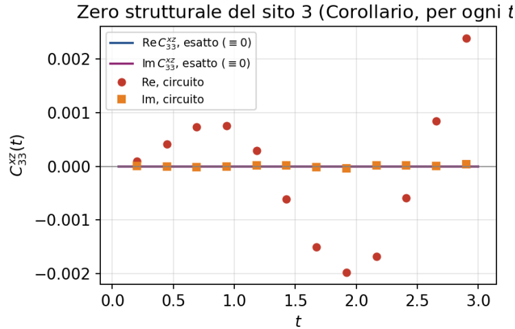
Figura 1: C_{33}^{xz}(t) : il calcolo classico esatto (linee, \equiv 0 per ogni t , Re e Im sovrapposte all'asse) confrontato con il circuito quantistico ( N = 200 passi di Trotter, punti). Zero strutturale per ogni t , non solo a t = 0 — conseguenza del sito 3 come punto fisso della simmetria residua U_{\text{anello}} , un tipo di zero che non può comparire nel dimero (dove ogni sito viene scambiato).
