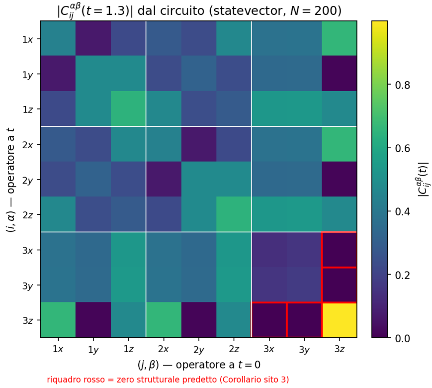
Figura 6: |C_{ij}^{\alpha\beta}(t=1.3)| per tutte le 81 combinazioni, misurato dal circuito (statevector, N=200 ). Righe e colonne raggruppate per sito (1, 2, 3), separatori bianchi fra i blocchi. I quattro riquadri rossi sono gli zeri strutturali del Corollario del sito 3 (Sez. 2.2): cadono esattamente dove previsto, dentro il blocco (3, 3).
