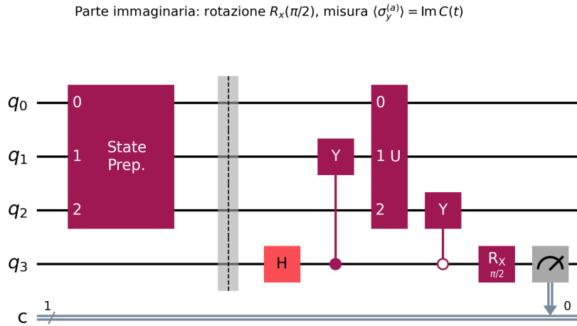
Figura 2: Le due esecuzioni del circuito per C_{12}^{yy}(t) : registro a 3 qubit ( q_0, q_1, q_2 ) più ancilla ( q_3 ). In entrambe: preparazione dello stato (box State Prep. ); Hadamard sull'ancilla; controlled- Y su q_1 = Q[2] (controllo pieno, W = \sigma_2^y ); blocco U(t) non controllato sui tre qubit di registro (box opaco — struttura interna in Sez. 6); anti-controlled- Y su q_2 = Q[1] (cerchio vuoto, V = \sigma_1^y ). Sopra : rotazione H e misura \Rightarrow \langle \sigma_x^{(a)} \rangle = \text{Re } C(t) . Sotto : rotazione R_x(\pi/2) e misura \Rightarrow \langle \sigma_y^{(a)} \rangle = \text{Im } C(t) .
