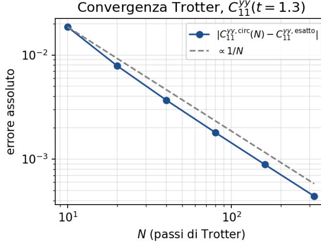
Figura 3: Errore del circuito rispetto al valore esatto, C_{11}^{yy}(t=1.3) , in funzione del numero di passi di Trotter N (scala doppio-logaritmica). La linea tratteggiata è 1/N . L'accordo con la pendenza attesa conferma che lo scarto residuo è solo errore di troncamento, malgrado la struttura a due livelli annidati discussa sopra: i livelli aggiuntivi cambiano il prefattore dell'errore, non il suo ordine in N .
