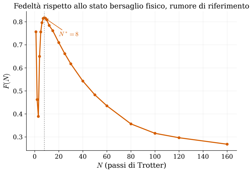
Figura 1: Fedeltà F(N) rispetto allo stato bersaglio fisico, in funzione del numero di passi di Trotter, a rumore di riferimento (ibm_torino). Crescita rapida per N piccolo (l'errore di Trotter domina), massimo a N^* = 8 , decrescita lenta per N grande (il rumore di gate accumulato domina).
