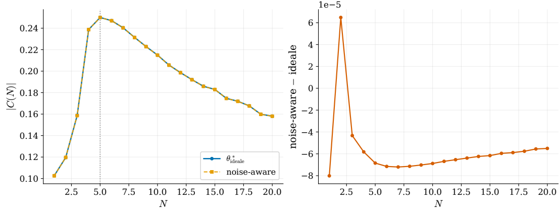
Figura 5: Sinistra: modulo del correlatore rumoroso, le due preparazioni a confronto — massimo a N^* = 5 in entrambi i casi. Destra: scostamento, scala ingrandita ( \sim 10^{-5} ) — un ordine di grandezza più piccolo persino dello scostamento osservato per la fedeltà di Trotter.
