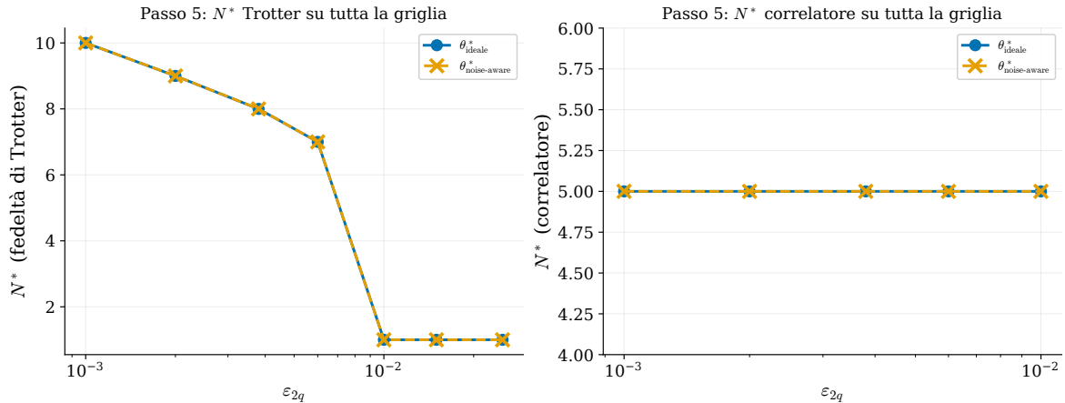
Figura 7: N^* in funzione di \varepsilon_{2q} , riuso ideale contro noise-aware, su tutta la griglia dello scan sui parametri di rumore. Sinistra: fedeltà di Trotter (con la nota transizione a N^* = 1 per rumore forte, già caratterizzata nello scan originale). Destra: modulo del correlatore. Le due curve sono sovrapposte in ogni punto.
