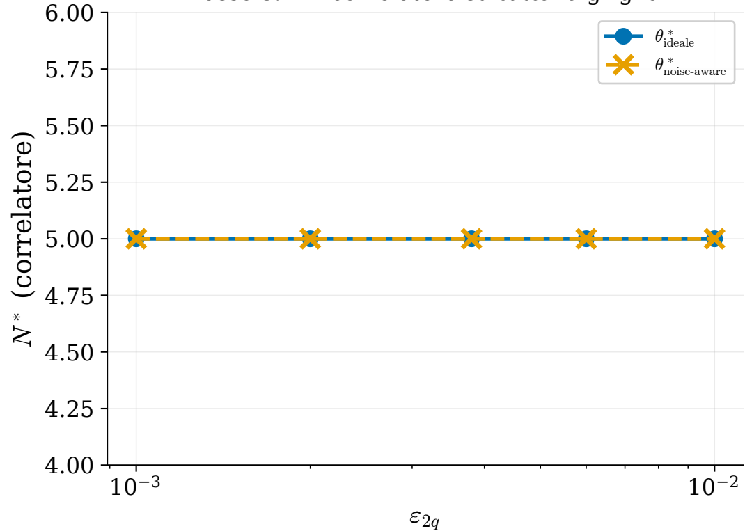
Passo 5: N^* correlatore su tutta la griglia
