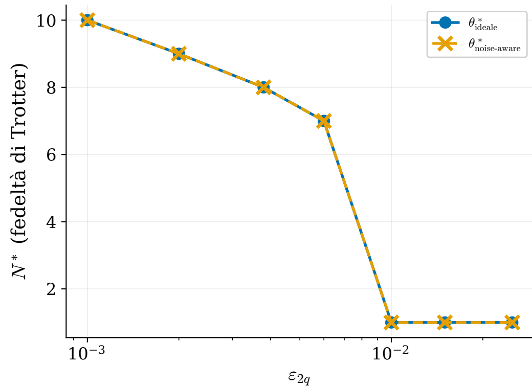
Passo 5: N^* Trotter su tutta la griglia
