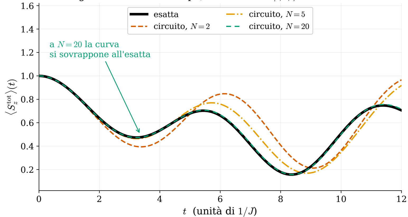
Magnetizzazione nel tempo, stato iniziale |\uparrow\uparrow\rangle --- circuito vero
