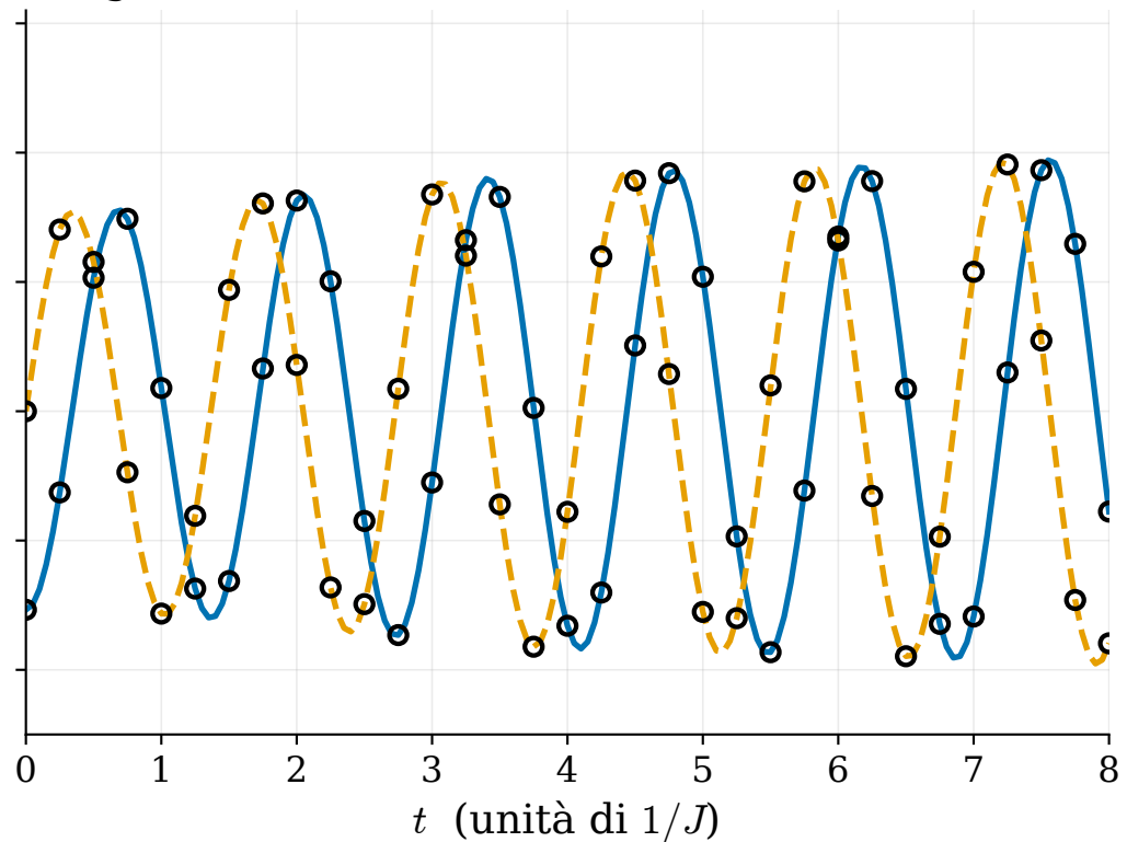
segnale monocromatico: scarto massimo 8.9e-15
