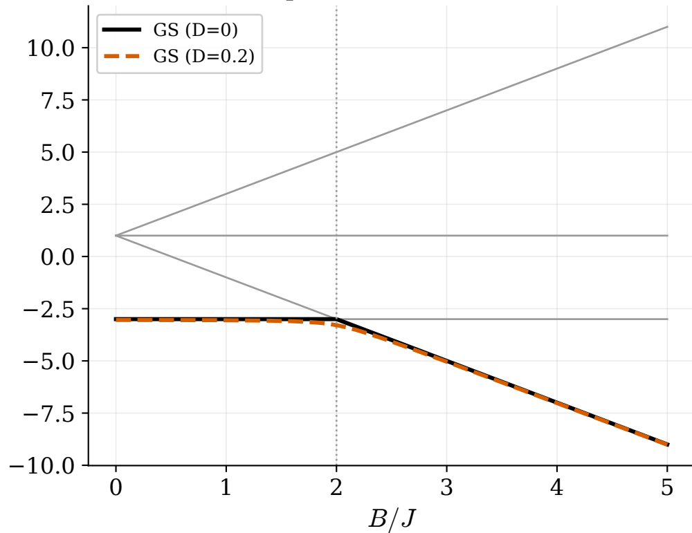
Spettro del dimero
