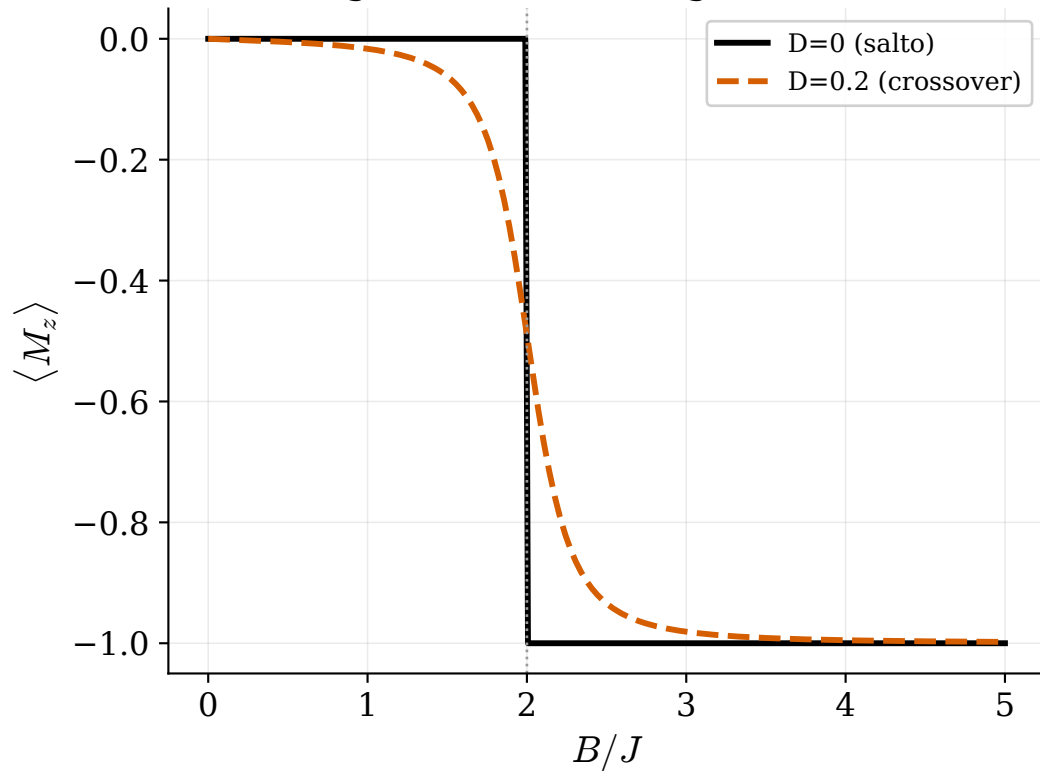
Magnetizzazione del ground state
