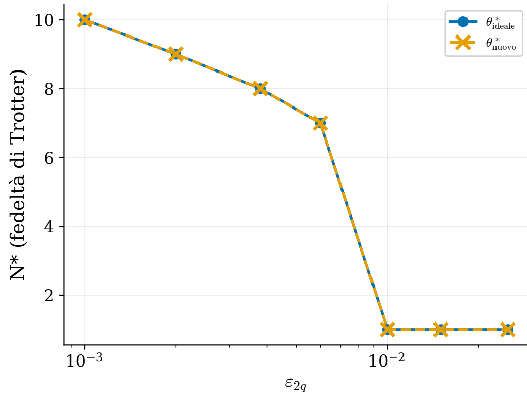
N* Trotter su tutta la griglia
