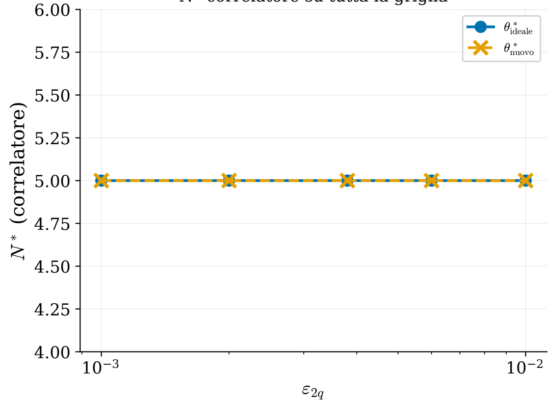
N* correlatore su tutta la griglia
