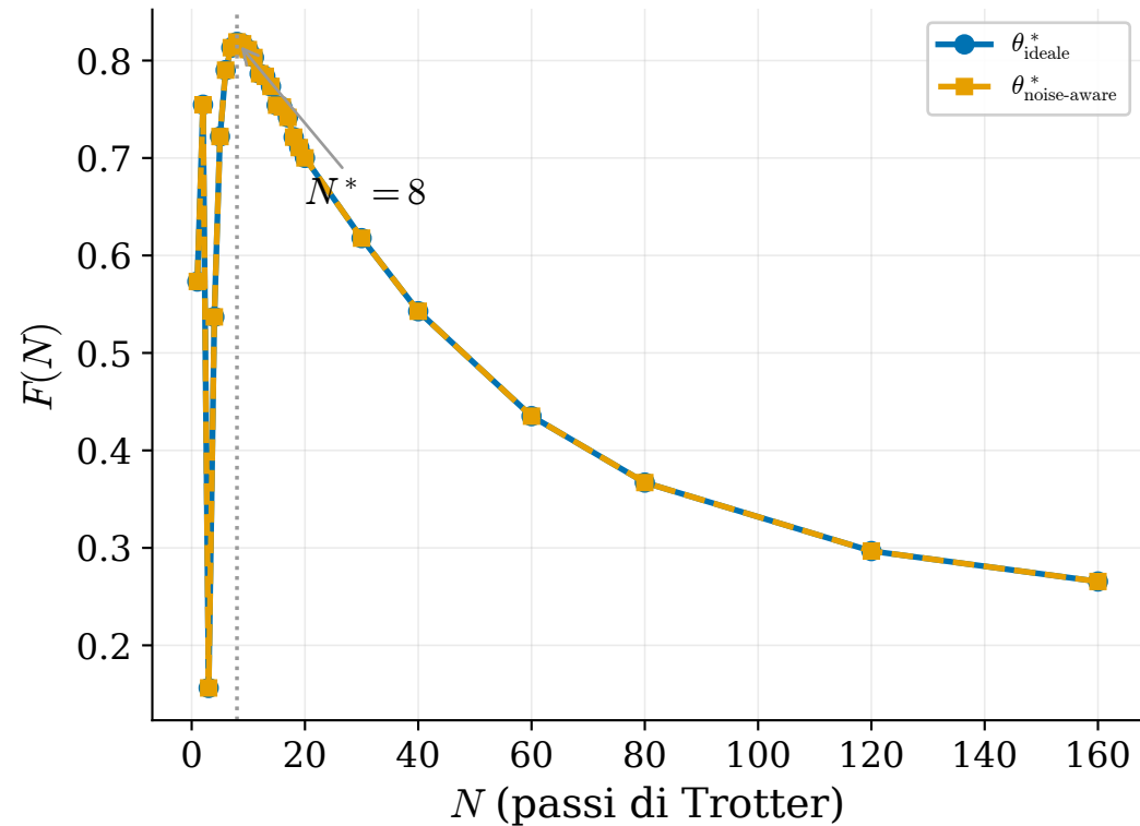
Fedeltà di Trotter (secondo punto)
