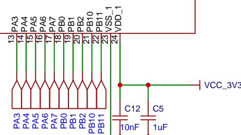
MCU最小系統
