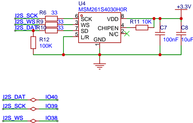
數字麥克風部分
