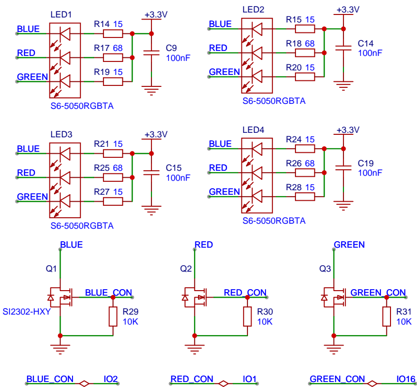
RGB三色燈部分
