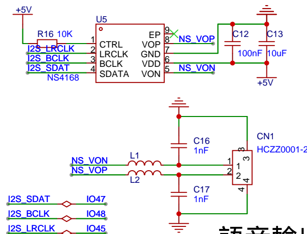
語音輸出部分
