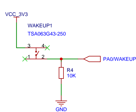
喚醒按鍵
