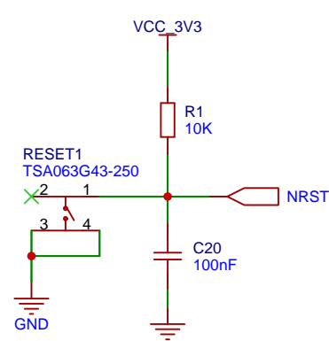
復位按鍵
