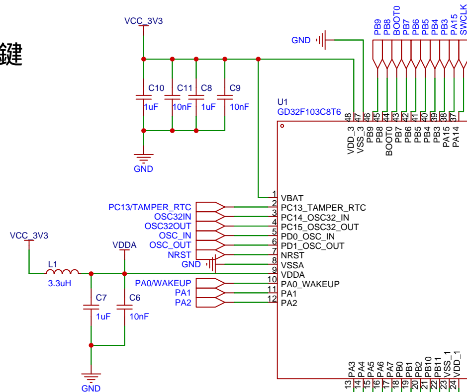
MCU最小系統
