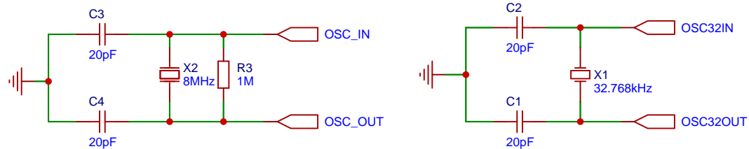
外部晶震
