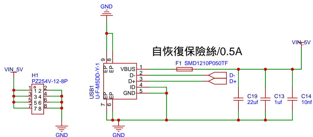
micro輸入口
