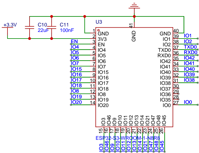
ESP32S3主控部分
