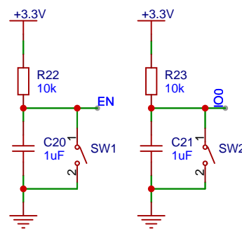
BOOT&復位按鍵部分
