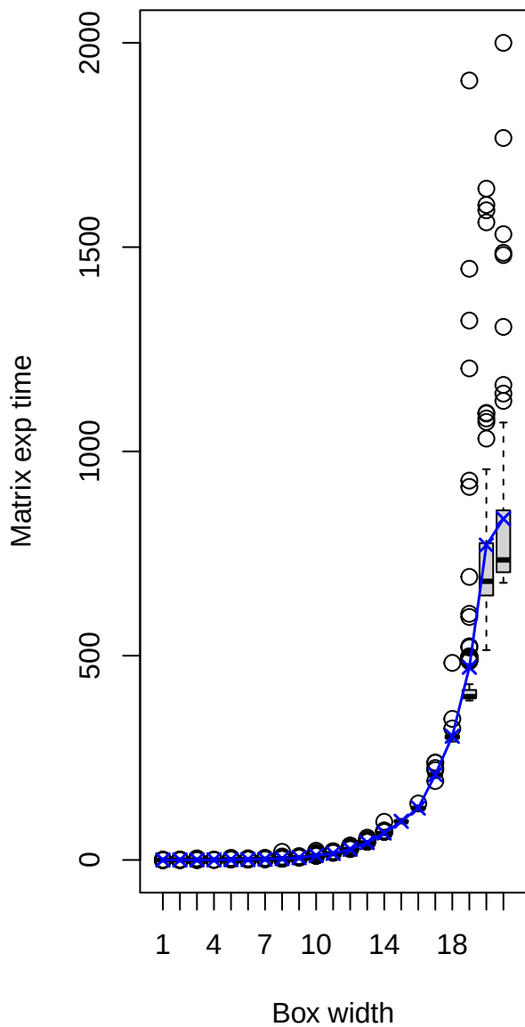
ARMA
