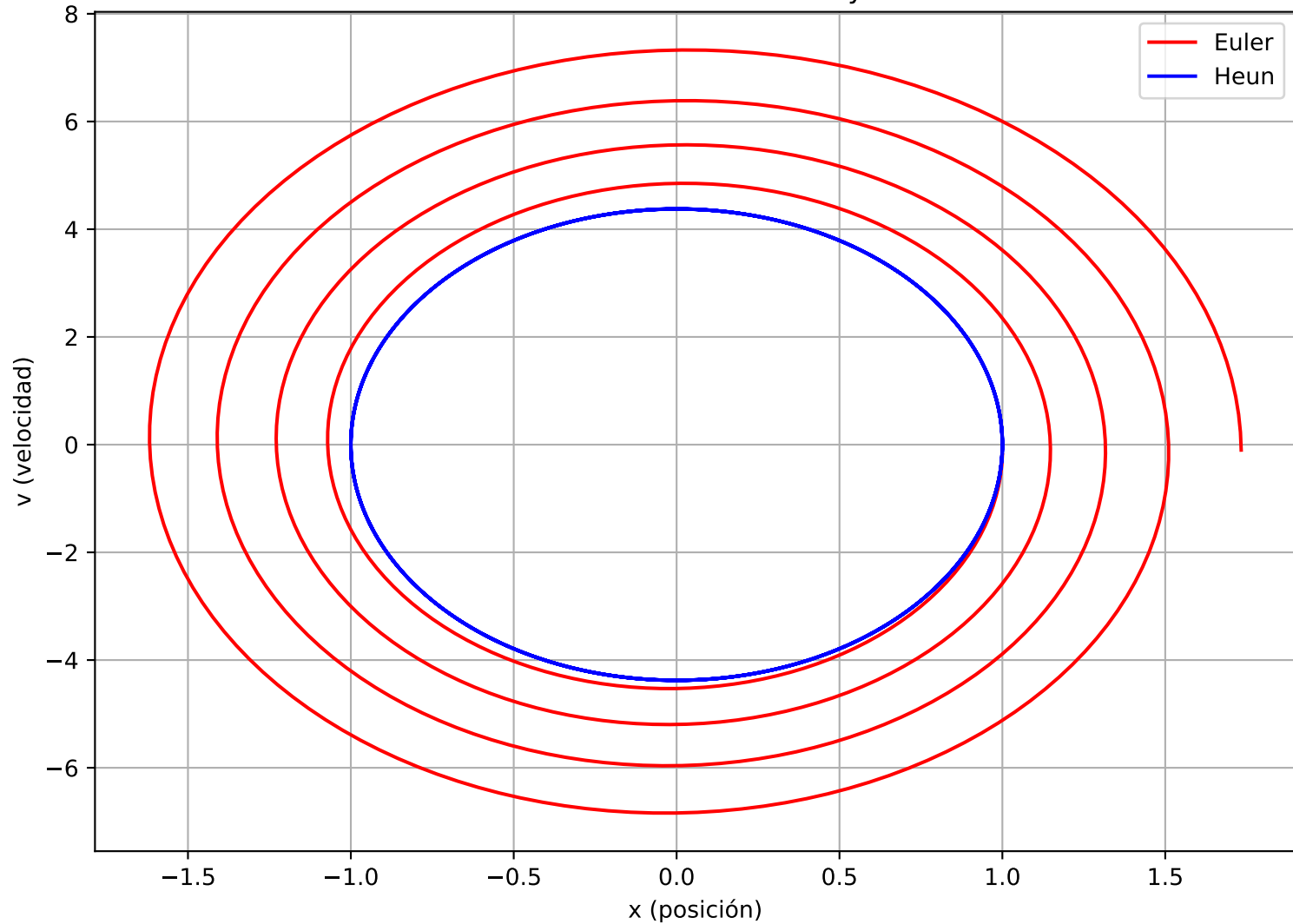
Velocidad vs Posición - Euler y Heun
