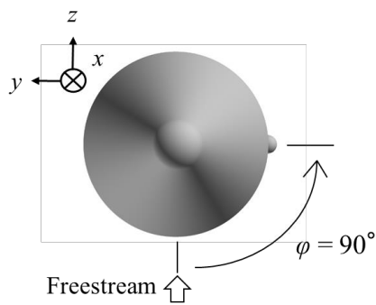
(d) Protuberance position (roll angle).
