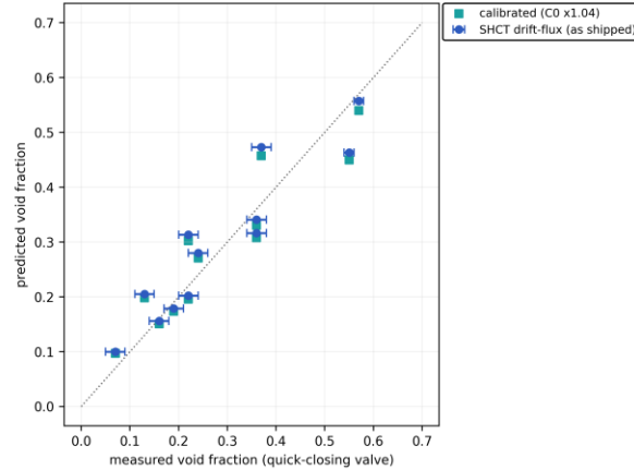
Flow-loop holdup validation vs LabPetro / CEPETRO, Universidade Estadual de Campinas (UNICAMP). Air-water, horizontal, 600 s per point.
