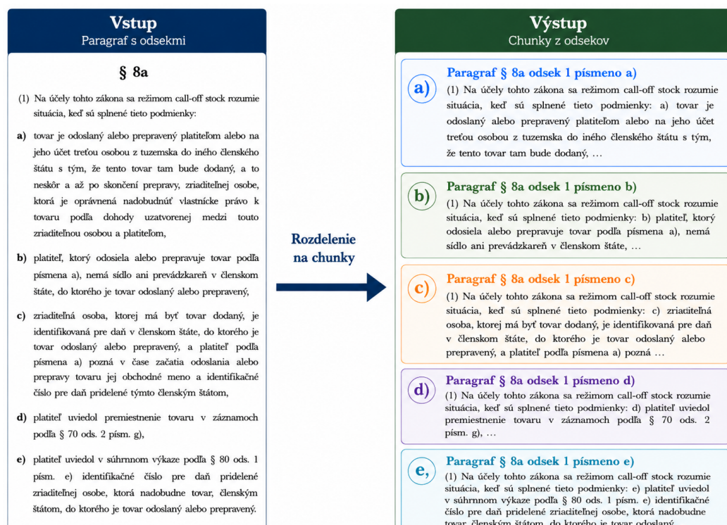
Obr. 11: Ukážka rozdelenia paragrafu slovenského zákona na chunky podľa hierarchickej štruktúry paragraf -> odsek -> písmeno -> bod. Každý chunk obsahuje text najhlbšej úrovne spolu s nadradeným kontextom paragrafu a odseku, aby bol čitateľný samostatne a zachoval si právny zmysel.
