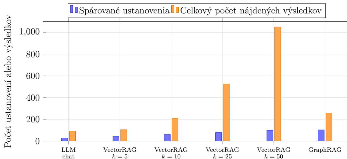
Obr. 13: Porovnanie počtu ustanovení spárovaných s ľudskou anotáciou a celkového počtu nájdených referencií alebo chunkov pre jednotlivé prístupy na testovacej množine 21 otázok, kde je počet hľadaných referencií 138.
