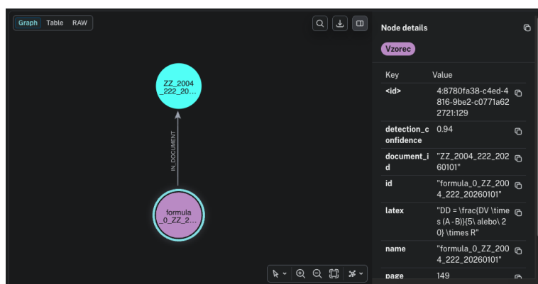
Obr. 4: Uzol typu Vzorec extrahovaný zo zákona o dani z pridanej hodnoty a jeho väzba IN_DOCUMENT na nadradený uzol dokumentu. Vo vlastnostiach uzla sa zachováva LaTeX prepis matematického zápisu, istota detekcie modelom DocLayout-YOLO a metaúdaje o zdroji (číslo strany, identifikátor dokumentu).
