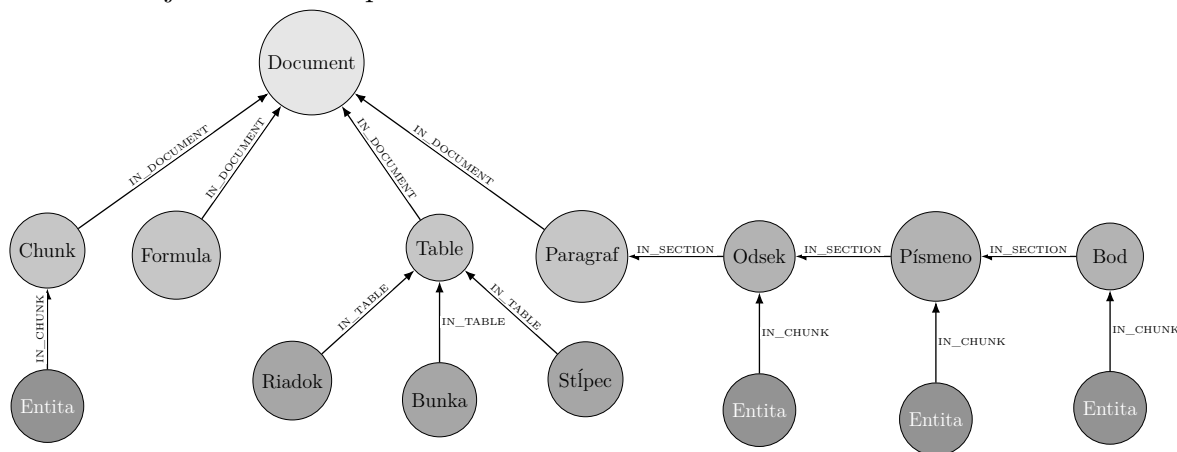
Obr. 7: Štruktúra znalostného grafu: dokument, obsahové uzly, hierarchia sekcií, entita a listy tabulky.
