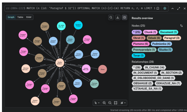
Obr. 8: Výsledok Cypher dotazu nad uzlom Paragraf § 32 zo zákona o DPH (222/2004 Z. z.) zobrazujúci všetkých susedov dostupných na jeden skok. Pravý panel sumarizuje rozloženie typov uzlov (Chunk, Odsek, Písmeno, Paragraf, Podmienka, Pravnypredpis, Sluzba, Tovar) a typov hrán (IN_DOCUMENT, IN_SECTION, OBSAHUJE, ODKAZUJE_NA, JE_OSLOBODENE_OD_DANE, VZTAHUJE_SA_NA).
