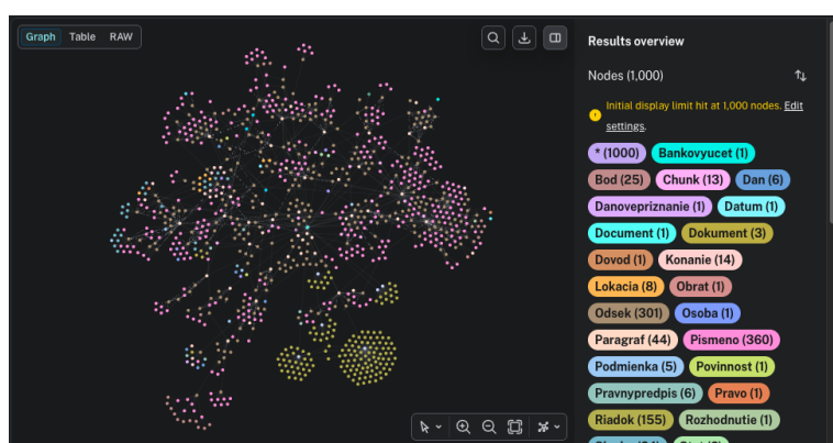
Obr. 9: Celkový pohľad na výsledný znalostný graf vybudovaný zo zákona o DPH obmedzený na 1000 uzlov.
