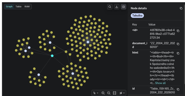
Obr. 3: Výsledok extrakcie tabuliek do znalostného grafu. Centrálne modré uzly predstavujú koreňové uzly typu Tabulka , žlté listové uzly sú jednotlivé riadky tabuľky obsahujúce vlastnosti stĺpcov. V pravom paneli sú zobrazené detaily vybraného uzla vrátane uchovaného HTML obsahu a väzby na zdrojový dokument.
