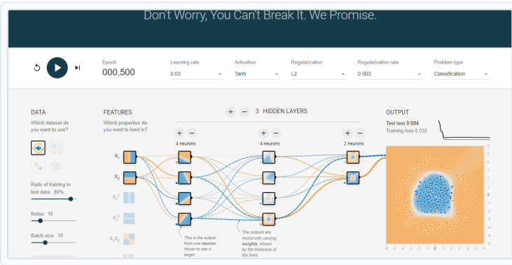
Figura 1. Captura de ejecución en TensorFlow Playground (Circle, L_2 , \alpha=0.03 , semilla 0.42, 500 épocas). Parámetros fijados en el panel DATA (split 80/20, ruido 10%, batch 10, red [4, 4, 2] con tanh) y superficie de separación concéntrica regular frente al ruido (test loss visible: 0.084, train loss: 0.032, 0/34 enlaces muertos).
