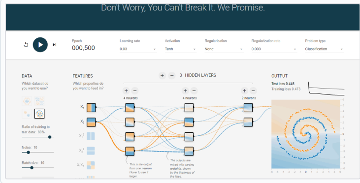
Figura 2. Captura de ejecución en TensorFlow Playground (Spiral, None, \alpha=0.03 , semilla s_1=0.42 , 500 épocas). Muestra la semilla s_1 , estancada casi sin separación efectiva entre clases (test loss: 0.445, train loss: 0.473). Con 34 pesos y coordenadas puras ( X_1, X_2 ), la red carece de capacidad inductiva para resolver las espirales.
