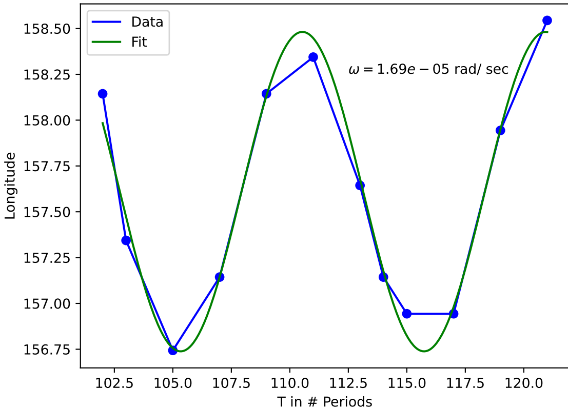
WS Longitude vs. Jupiter Periods
